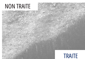
Surface émaillée non traitée et surface traitée avec Resin PoliStrip 15µm Agrandissement MeB 500x
