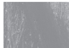
Surface émaillée traitée (40µm) et centre traité avec Resin PoliStrip Agrandissement SeM 15µm 2000x
